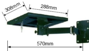
TTV-007 (12" ~ 14") • Max. Load : 30 kgs • Wall Mount w/Key Lock
