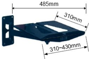
TTV-004A (14" ~18") • Max. Load : 30 kgs • Wall Mount Type
