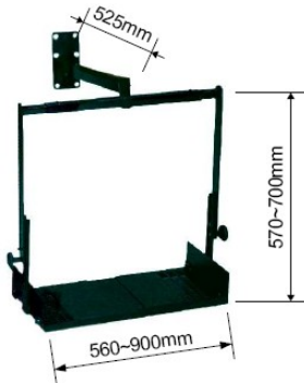
TTV-033A (20" ~29") • Max. Load : 75 kgs • Wall Mount Type
