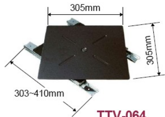
TTV-064 • TV Turntable • 電視機轉盤
