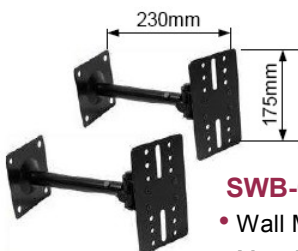
SWB-001 (喇叭支架) • Wall Mount Type • Max. Load : 10 kgs
