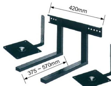
TTV-008 (音響 / 喇叭支架) • Hi-Fi & Speaker Bracket • Max. Load : 30 kgs
