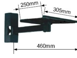
TTV-068A (9" ~12") • Max. Load : 30 kgs • Wall Mount Type
