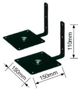
SP-007A (喇叭支架) • Wall Mount Type • Max. Load : 15 kgs
