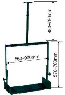
TTV-033 (20" ~29") • Max. Load : 75 kgs • Ceiling Mount Type
